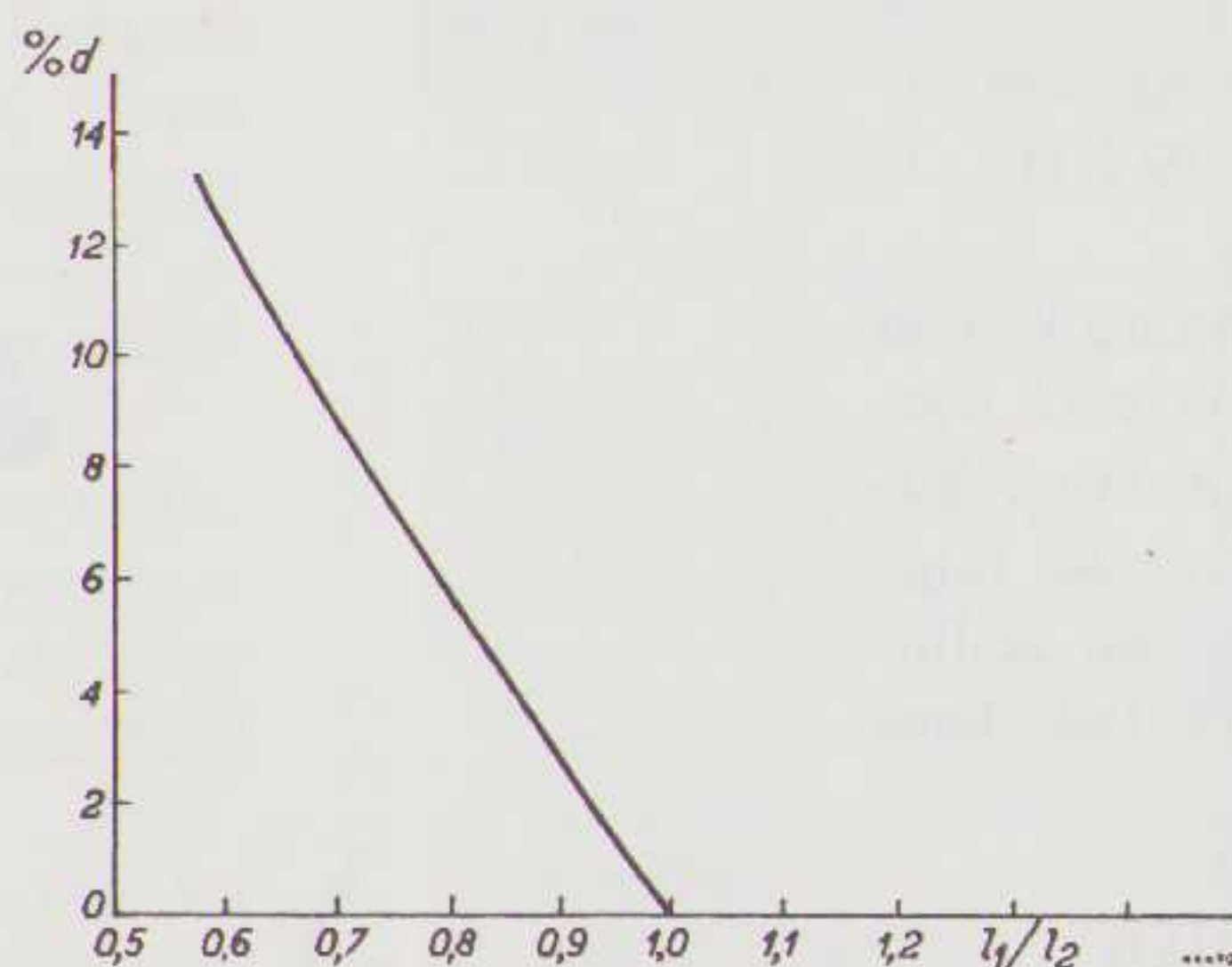
Fig. 3, Relatie tussen de verhouding I1-I2 en de vervorming
